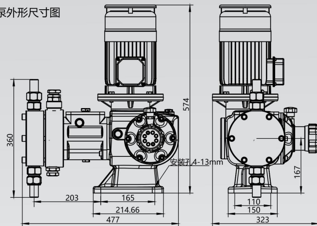
SDP-YB液压隔膜计量泵外形尺寸图
