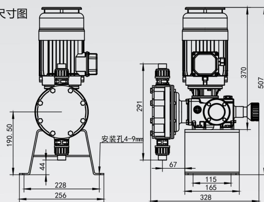
HK-A/B机械隔膜计量泵外形尺寸图
