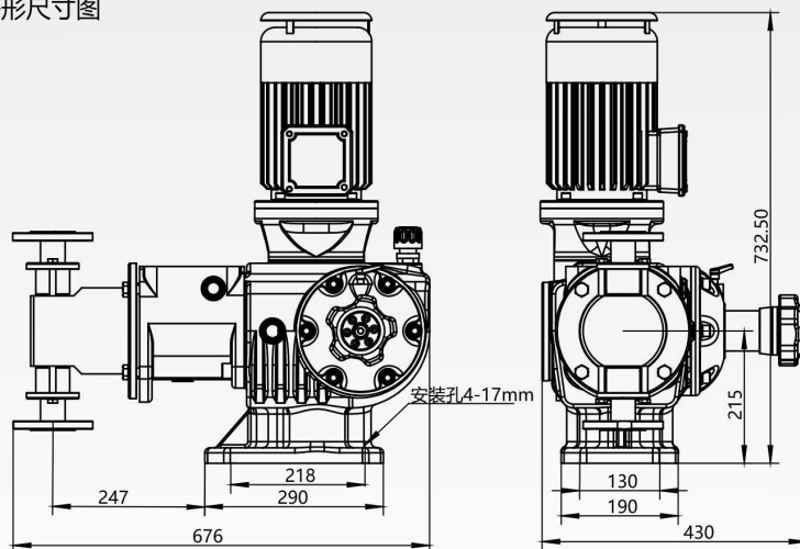
HZ-B柱塞计量泵外形尺寸图
