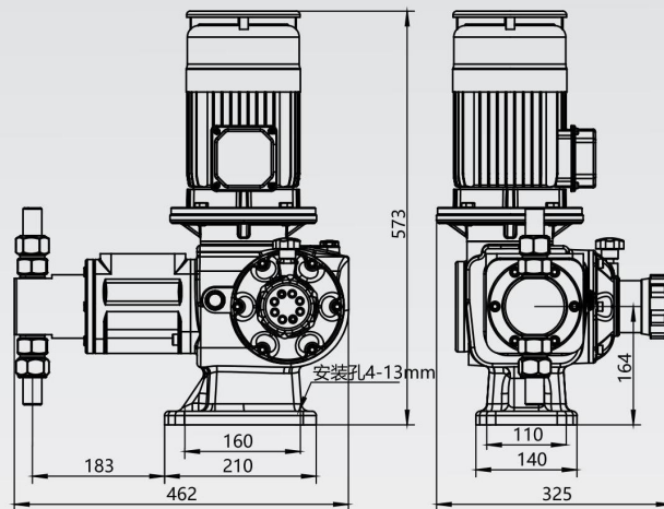
HZ柱塞计量泵外形尺寸图
