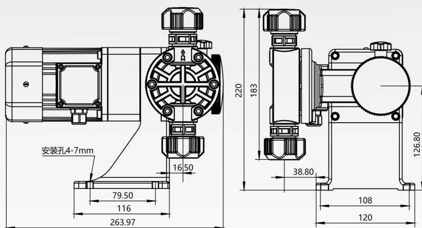
HL机械隔膜计量泵外形尺寸图
