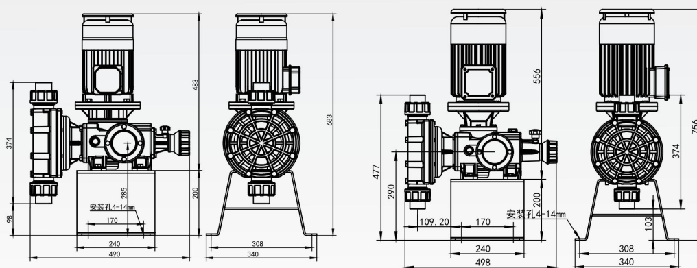
HK-A/B机械隔膜计量泵外形尺寸图
