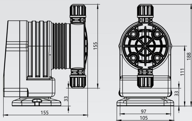
SDP-E电磁隔膜计量泵外形尺寸图
