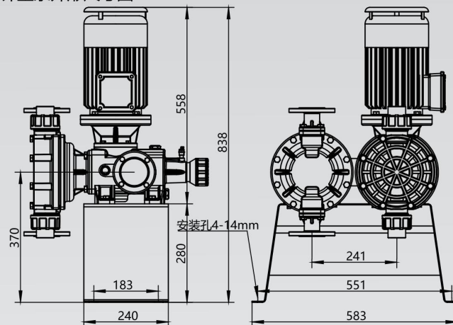
CT/HK-BX2-2000/1500多头计量泵外形尺寸图
