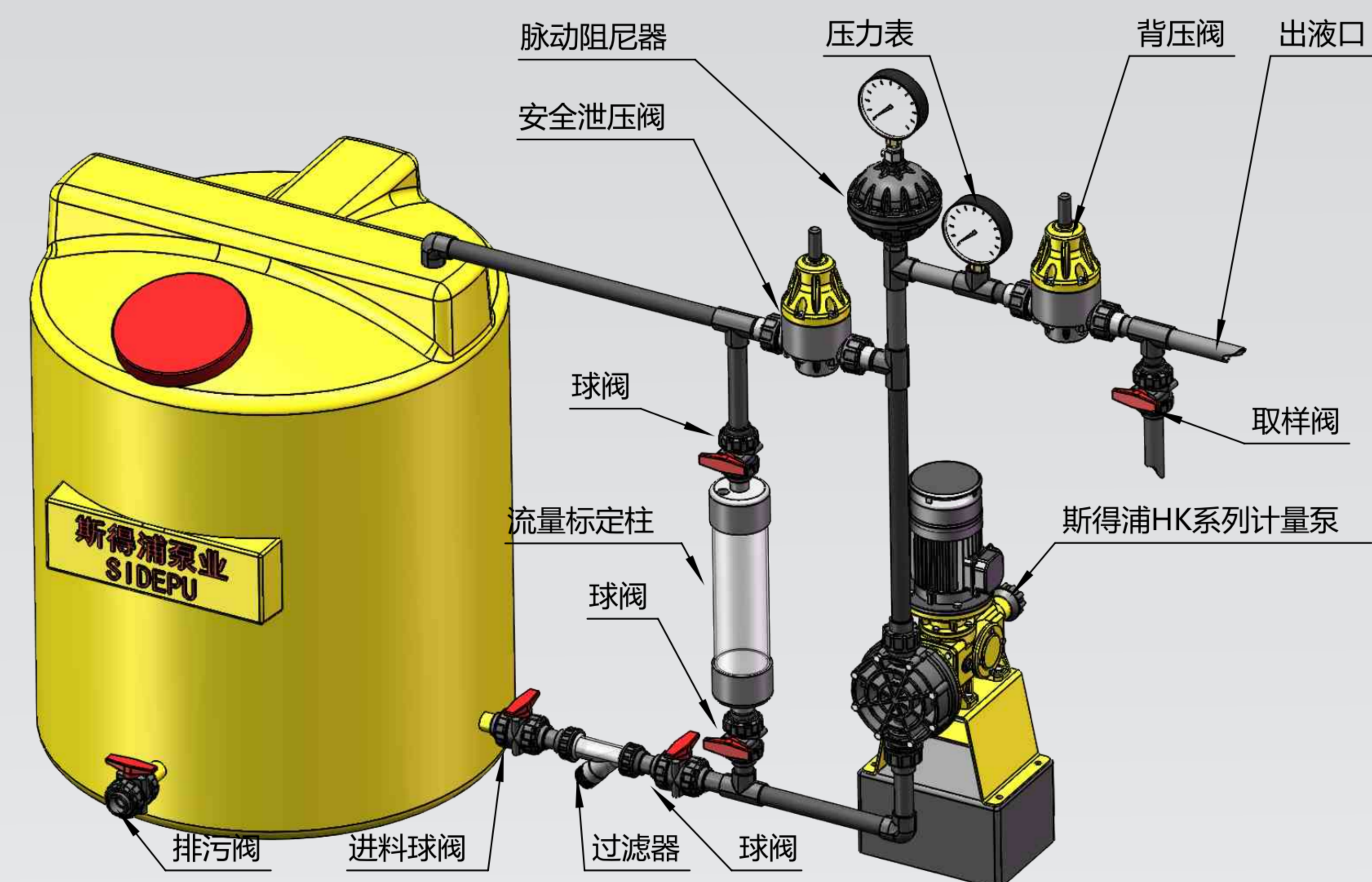
浸罐式管路系统安装示意图
