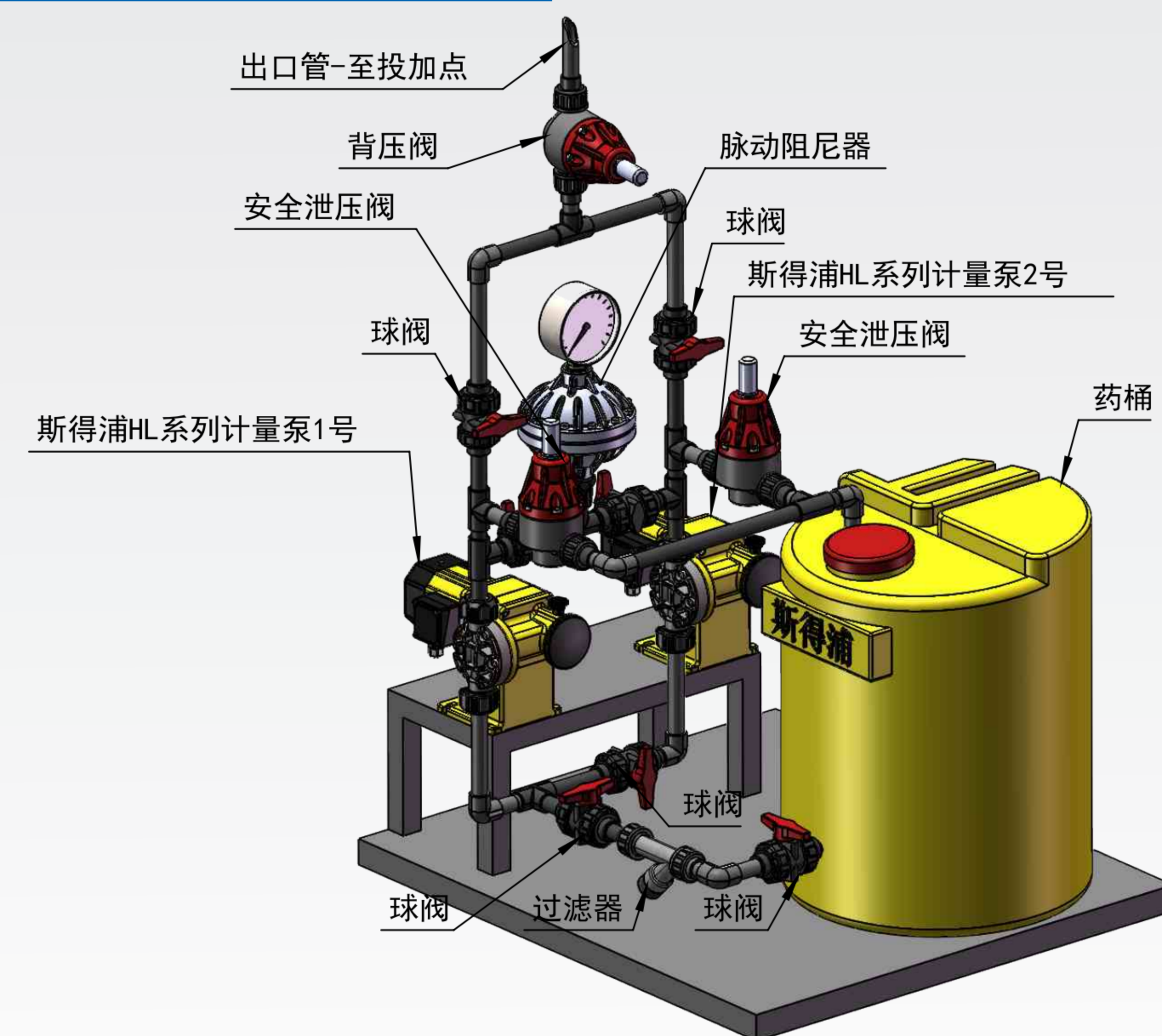
斯得浦计量泵一用一备加药系统安装示意图
